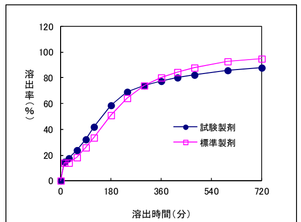
図9 pH7.5(200rpm)における平均溶出率
